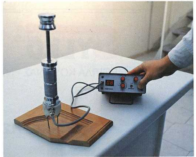
Μέτρηση της υγρασίας του ξύλου.
